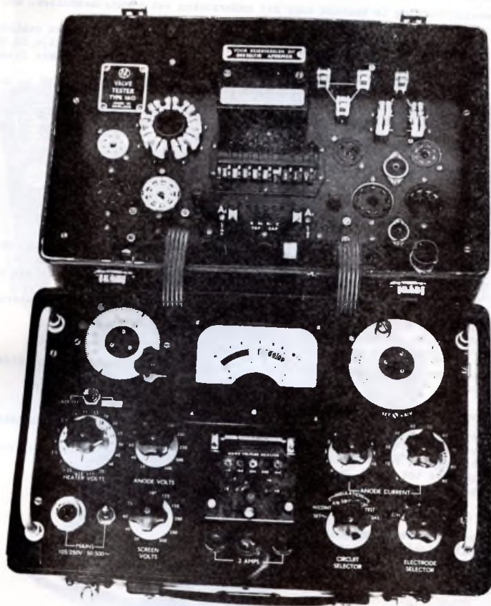
Fig 2 Bedieningspanelen van de meetuitrusting
