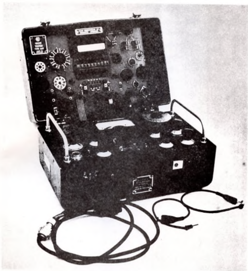
Fig 1 Meetuitrusting, elektronenbuis TV-3001/U
