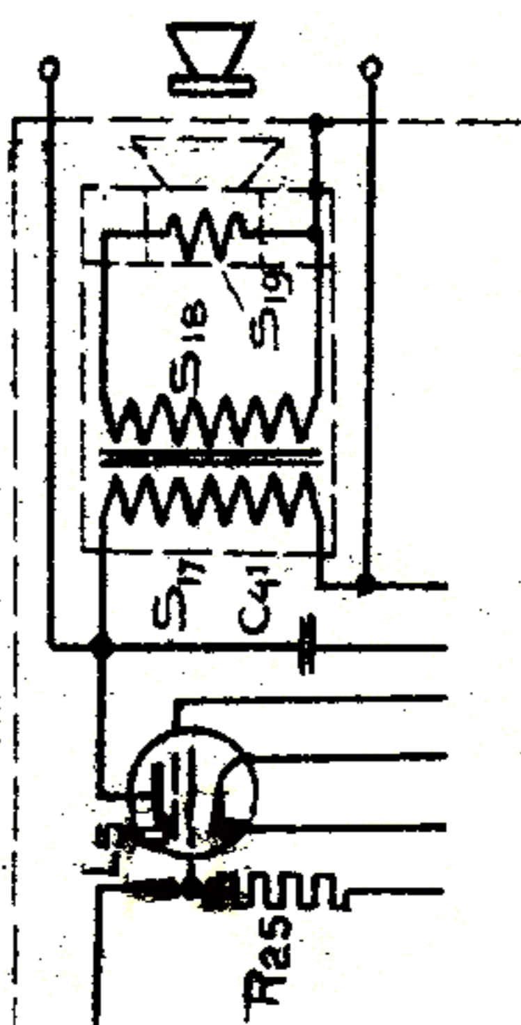
Uitv. RADIOKAST 730 A.
