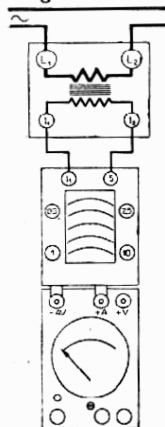
Stromwandler. Abb. 4
